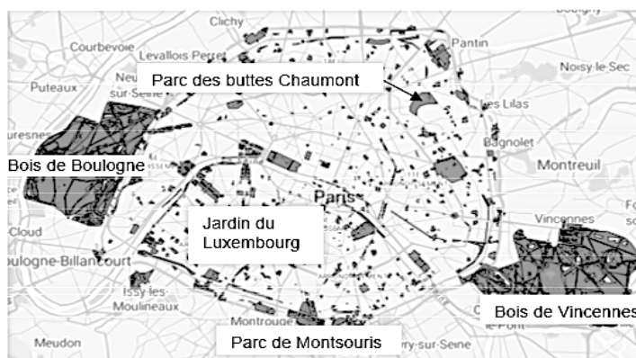
Figure C – Plan de localisation des îlots de fraîcheur dans Paris
